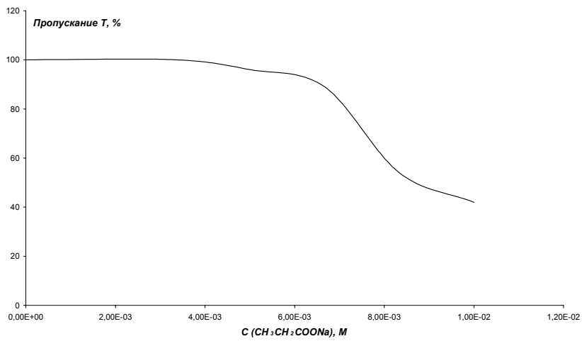
Зависимость мутности золя от концентрации электролита
