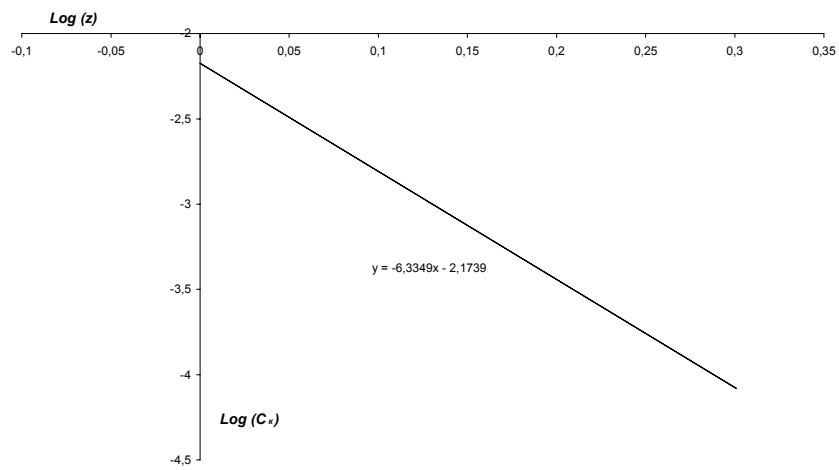
Зависимость порога коагуляции от валентности противоионов
